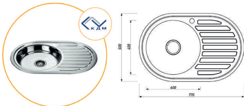
МОЙКА ОВАЛЬНАЯ (ЛЕВАЯ)
