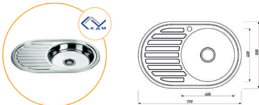
МОЙКА ОВАЛЬНАЯ (ПРАВАЯ)
